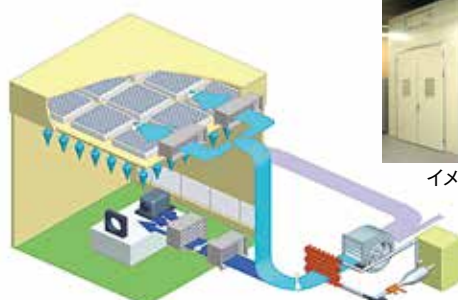
精密環境チャンバ システム概念
